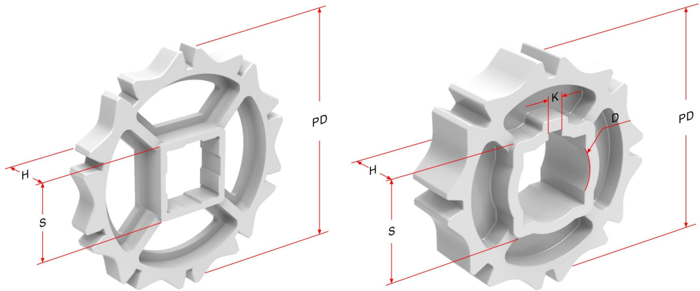
Sprocket Dimensions
