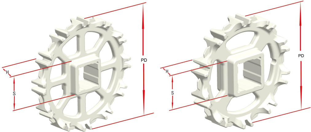
Sprocket Dimensions
