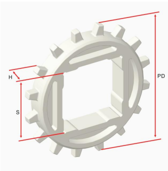
Sprocket Dimensions
